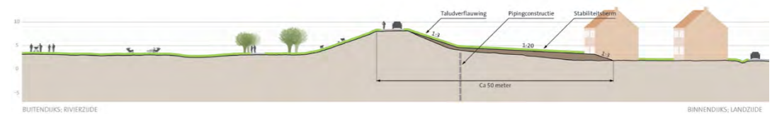
profiel dijkvak 3c
