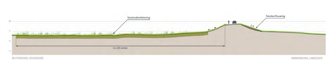
profiel dijkvak 5a
