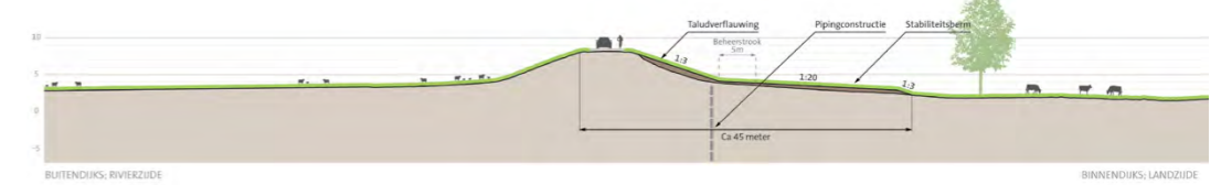
profiel dijkvak 3a
