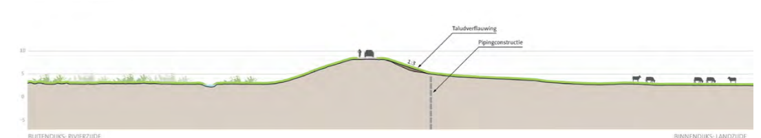
profiel dijkvak 5b
