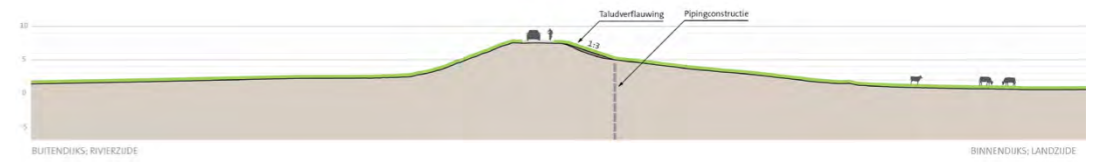
profiel dijkvak 2c
