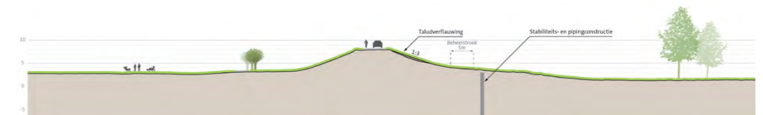
profiel dijkvak 3c
