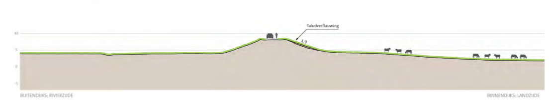
profiel dijkvak 4b
