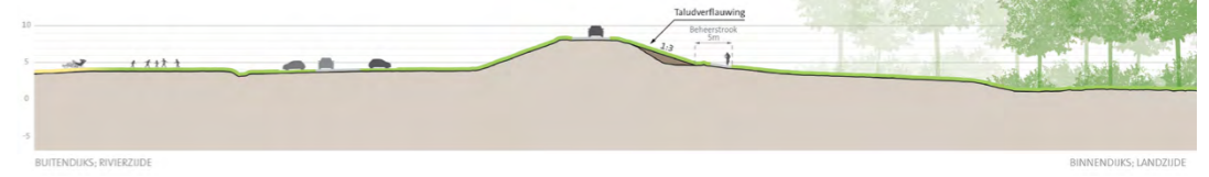
profiel dijkvak 4a
