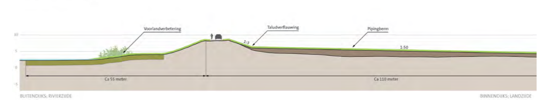
profiel dijkvak 4c
