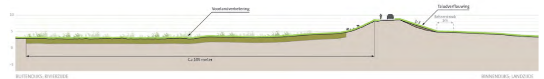
profiel dijkvak 5b - optie 1
