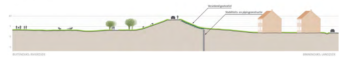
profiel dijkvak 3c
