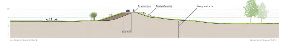
profiel dijkvak 3d
