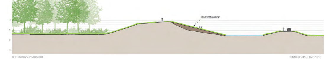
profiel dijkvak 9c
