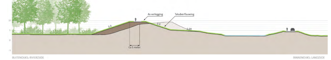
profiel dijkvak 9c
