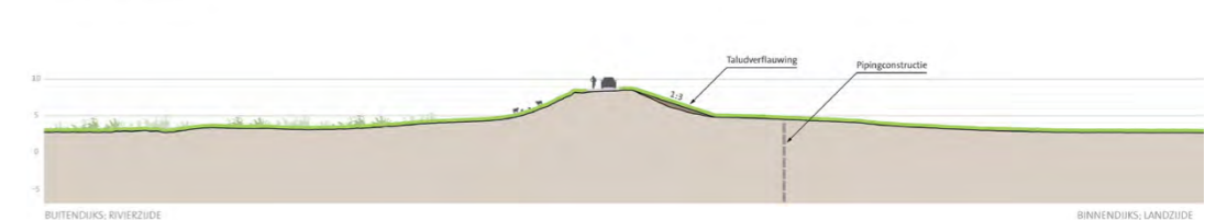
profiel dijkvak 5a
