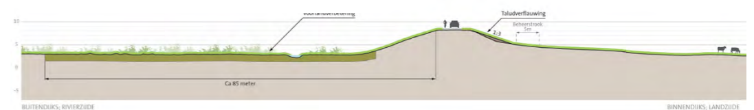
profiel dijkvak 9c
