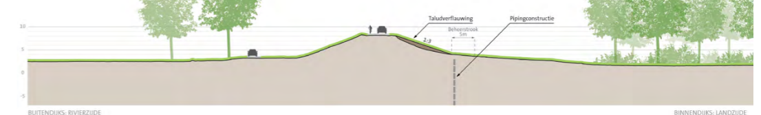
profiel dijkvak 3d
