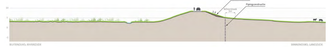
profiel dijkvak 5b - optie 2
