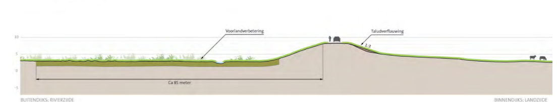
profiel dijkvak 5b
