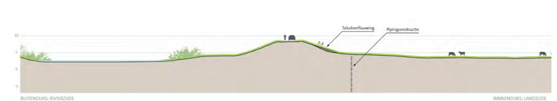
profiel dijkvak 4c
