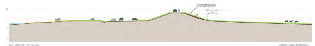
profiel dijkvak 4b
