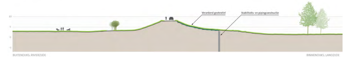
profiel dijkvak 3d
