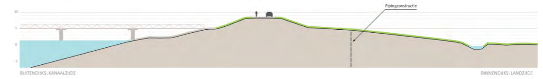
profiel dijkvak 2a
