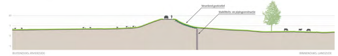
profiel dijkvak 3a
