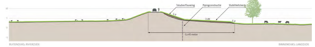
profiel dijkvak 3a
