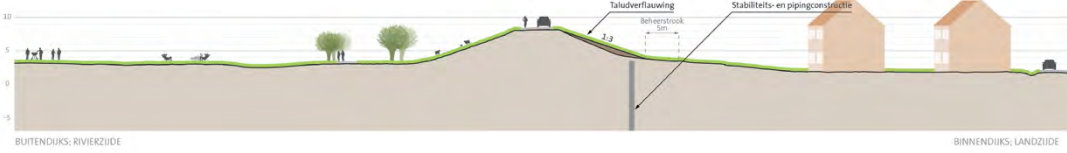
profiel dijkvak 3c
