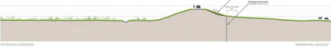
profiel dijkvak 5b - optie 2
