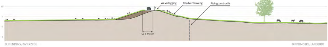
profiel dijkvak 3a
