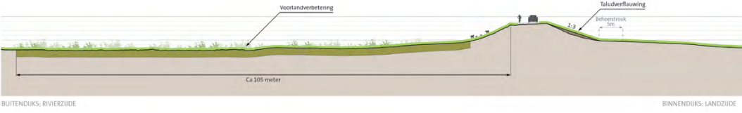
profiel dijkvak 5b - optie 1
