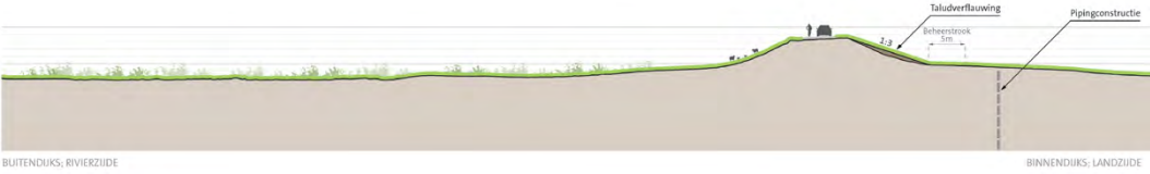
profiel dijkvak 5a - optie 2
