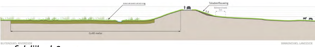
profiel dijkvak 9c
