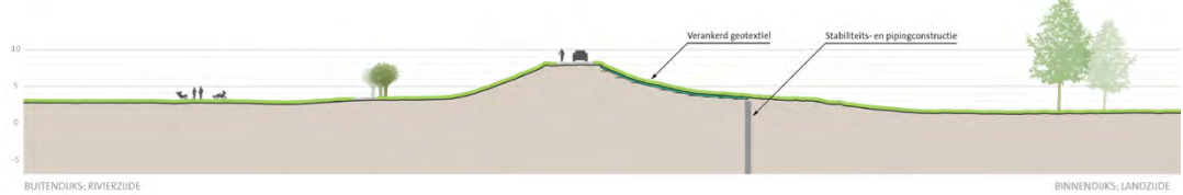
profiel dijkvak 3d
