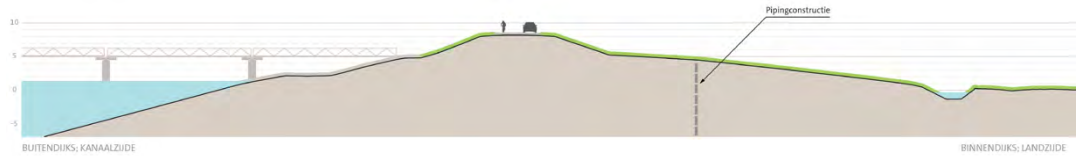
profiel dijkvak 2a
