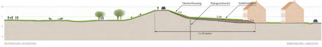
profiel dijkvak 3c
