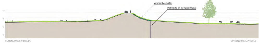
profiel dijkvak 3a
