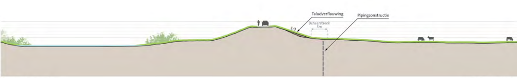
profiel dijkvak 5a - optie 1
