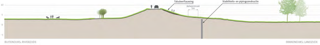
profiel dijkvak 3d
